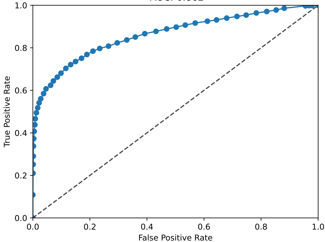
ZBTB20 ROC Curve AUC: 0.862
