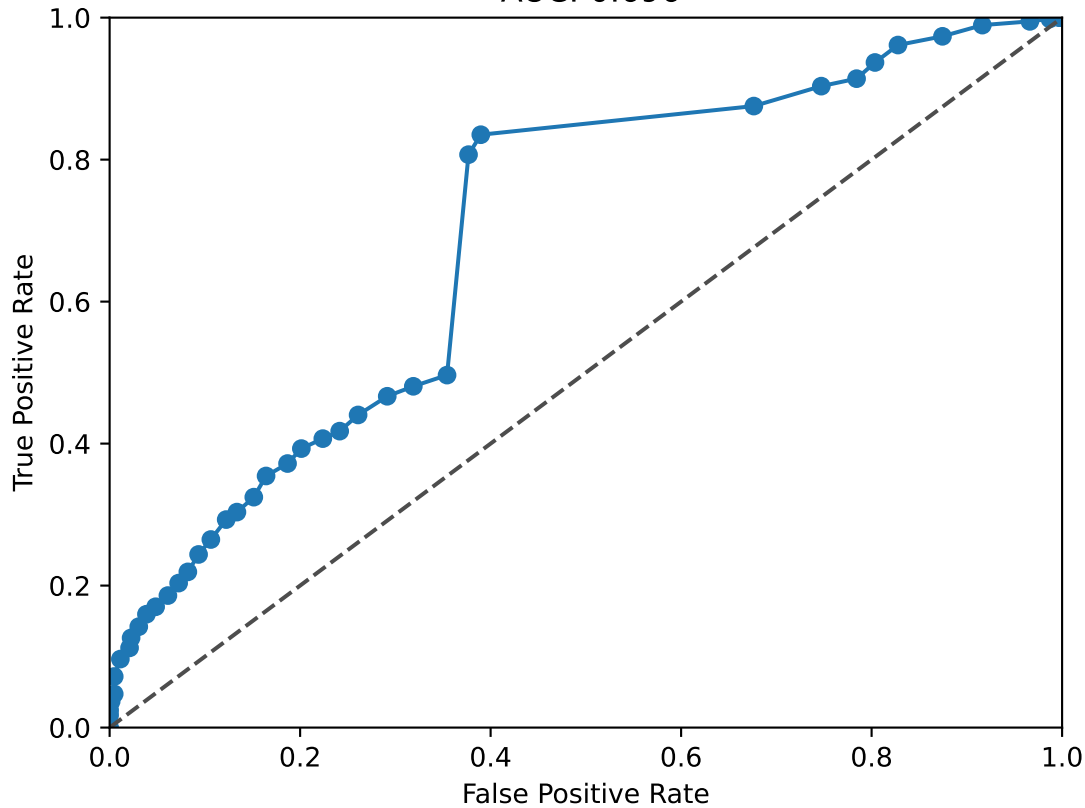
BACH2 ROC Curve AUC: 0.696
