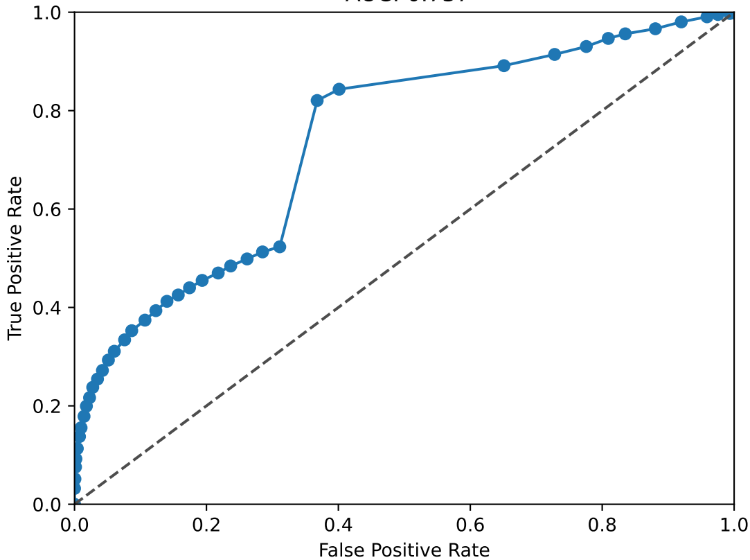
BACH2 ROC Curve AUC: 0.737
