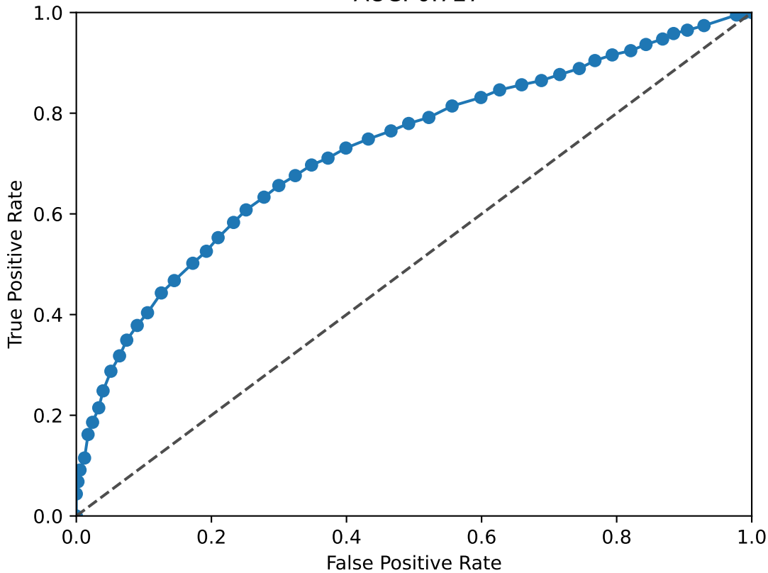
ZBTB20 ROC Curve AUC: 0.727
