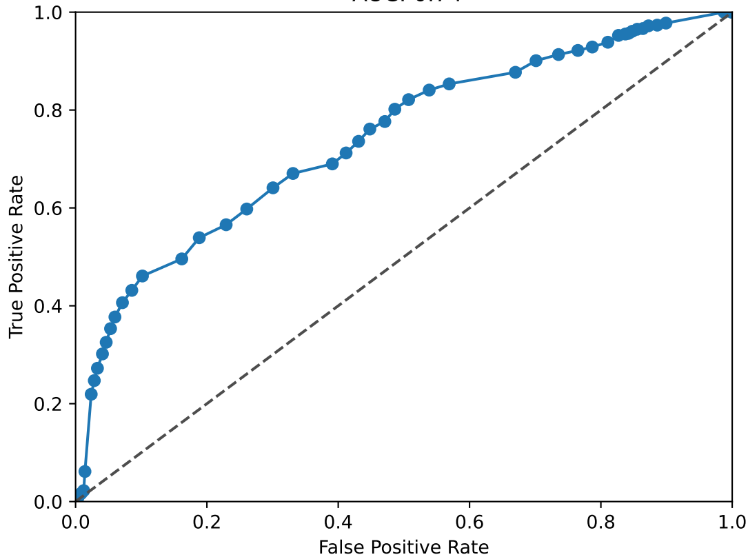
LMX1B ROC Curve AUC: 0.74
