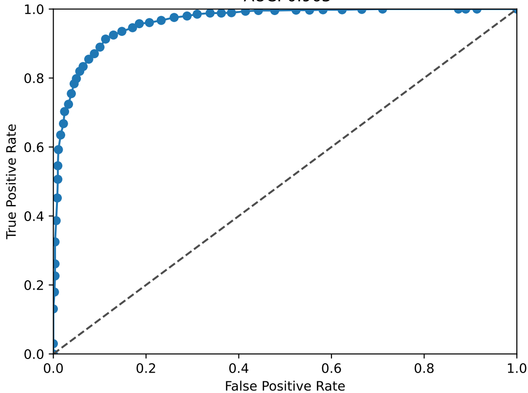
ZBTB20 ROC Curve AUC: 0.963
