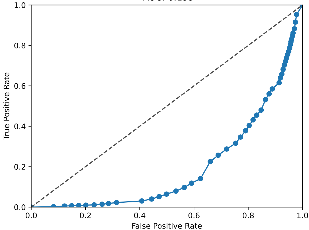
MEIS2 ROC Curve AUC: 0.199
