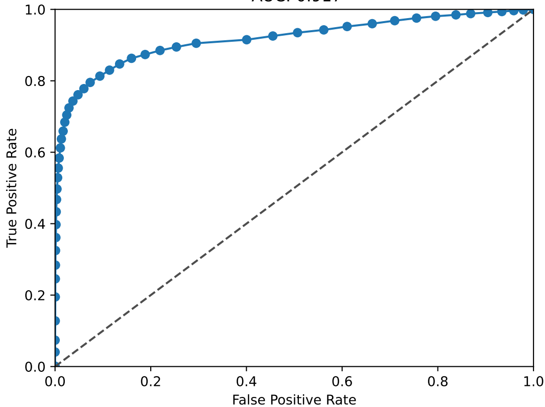
ZBTB20 ROC Curve AUC: 0.917
