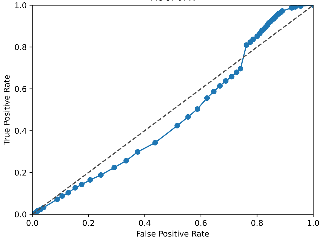
MEIS2 ROC Curve AUC: 0.47
