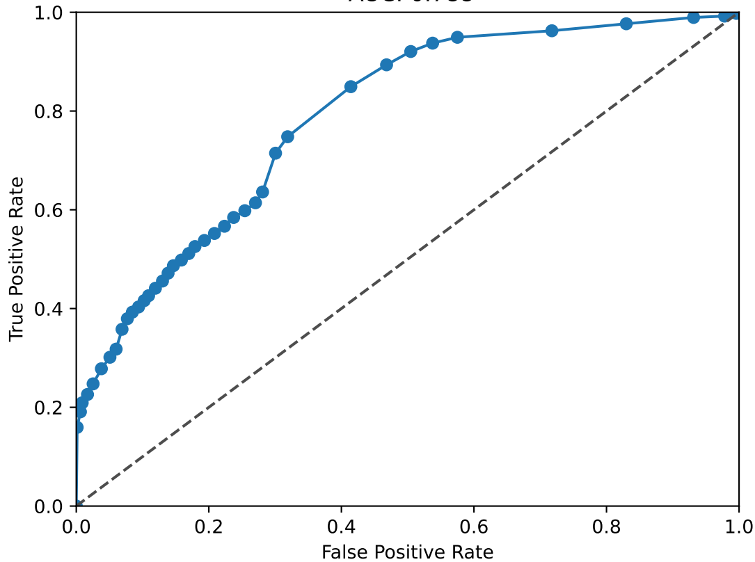
BACH2 ROC Curve AUC: 0.788
