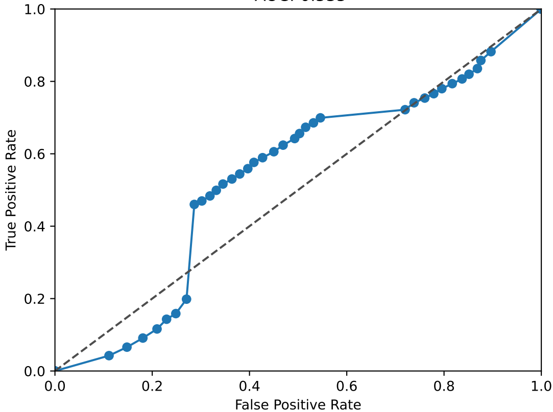
EHF ROC Curve AUC: 0.535
