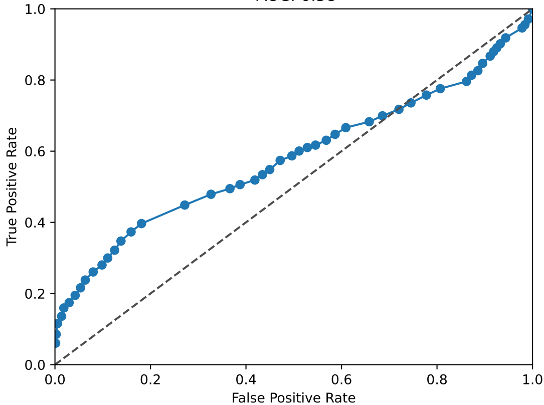
LMX1B ROC Curve AUC: 0.58
