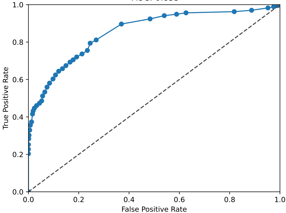
BACH2 ROC Curve AUC: 0.855
