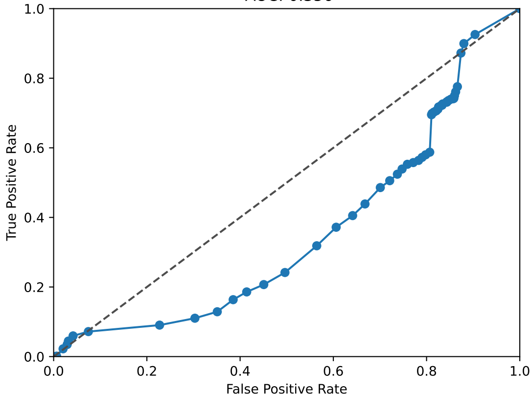
MEIS2 ROC Curve AUC: 0.356
