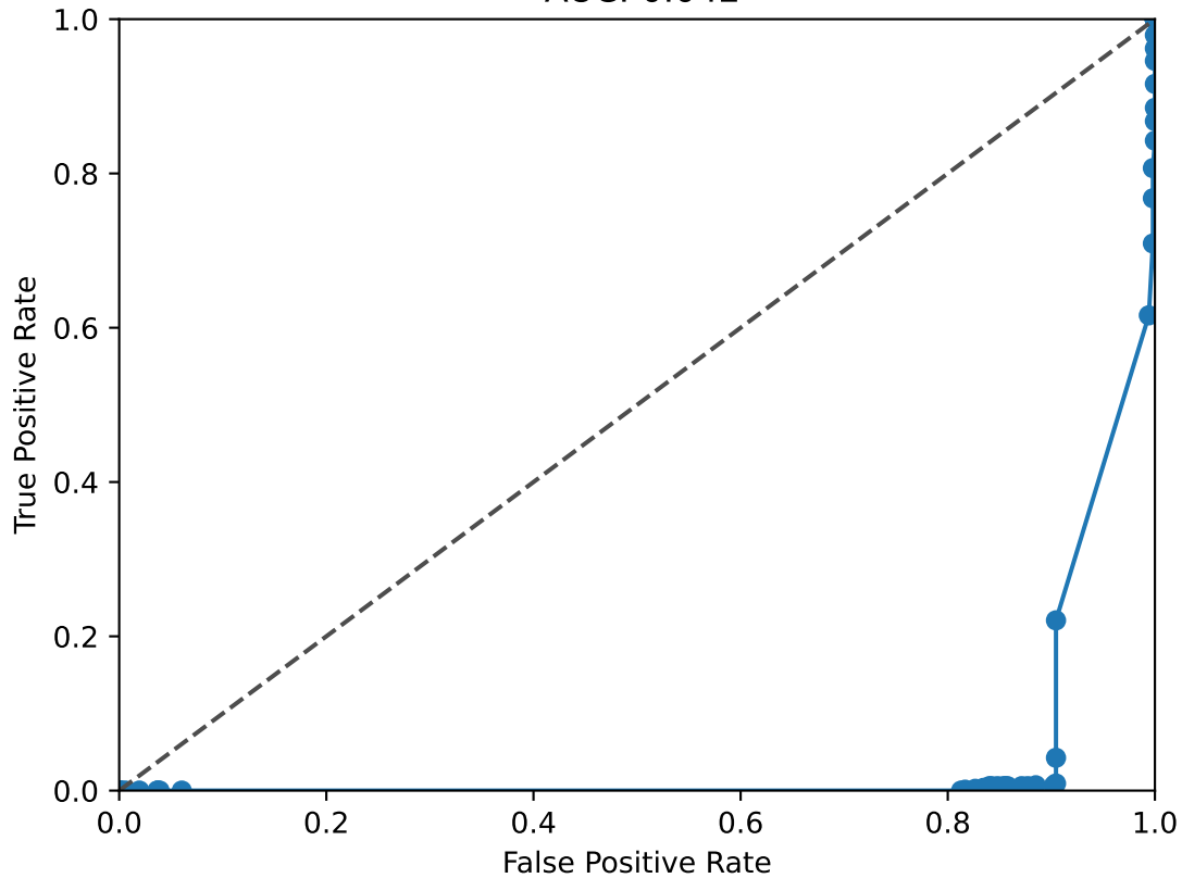
EHF ROC Curve AUC: 0.042
