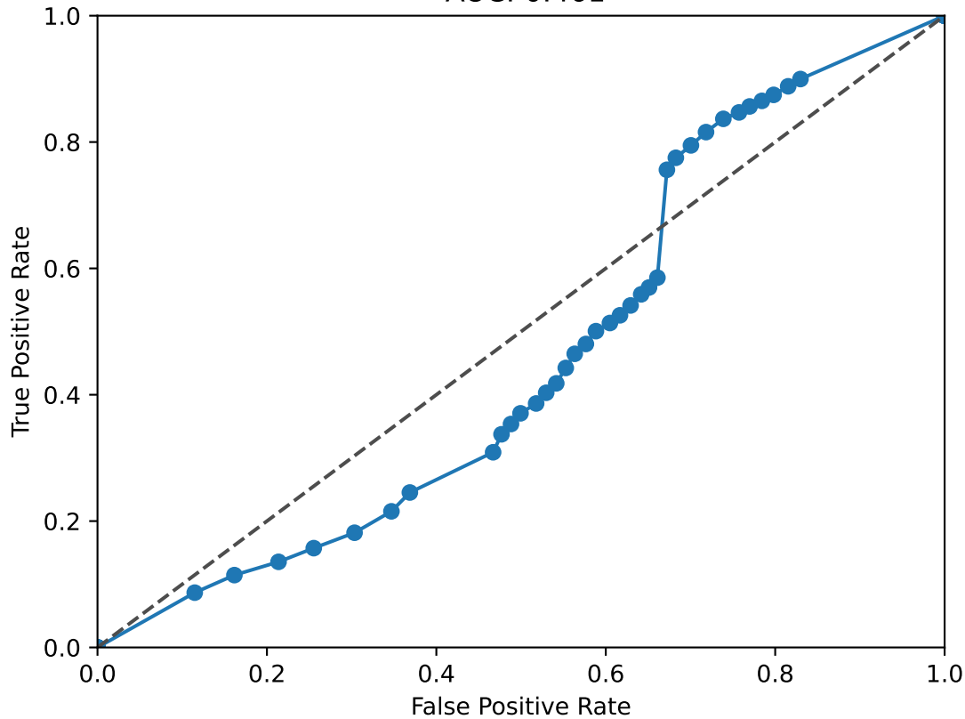
EHF ROC Curve AUC: 0.461
