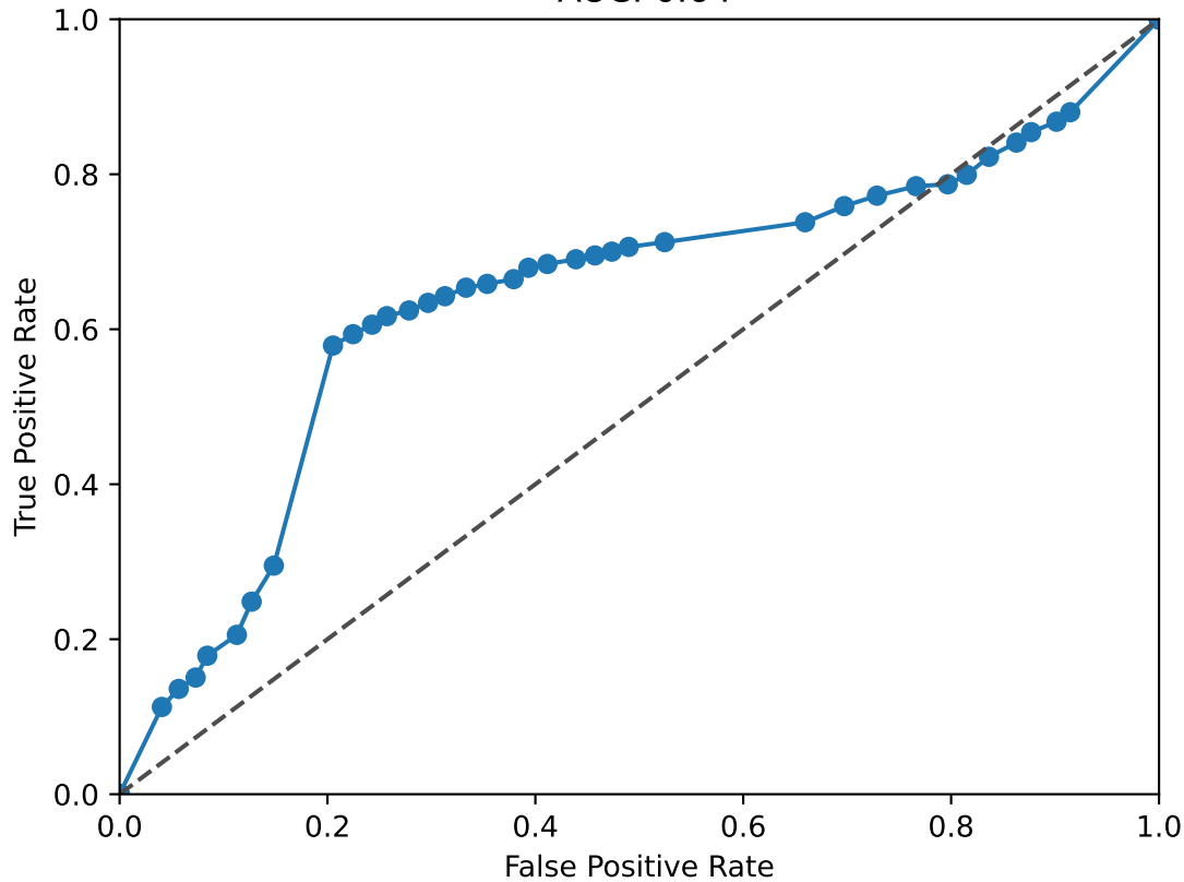
EHF ROC Curve AUC: 0.64
