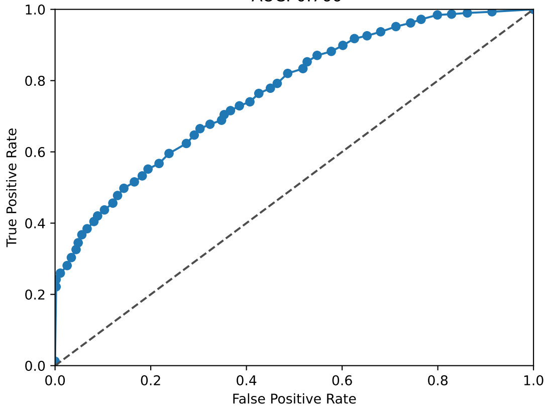
ZBTB20 ROC Curve AUC: 0.766
