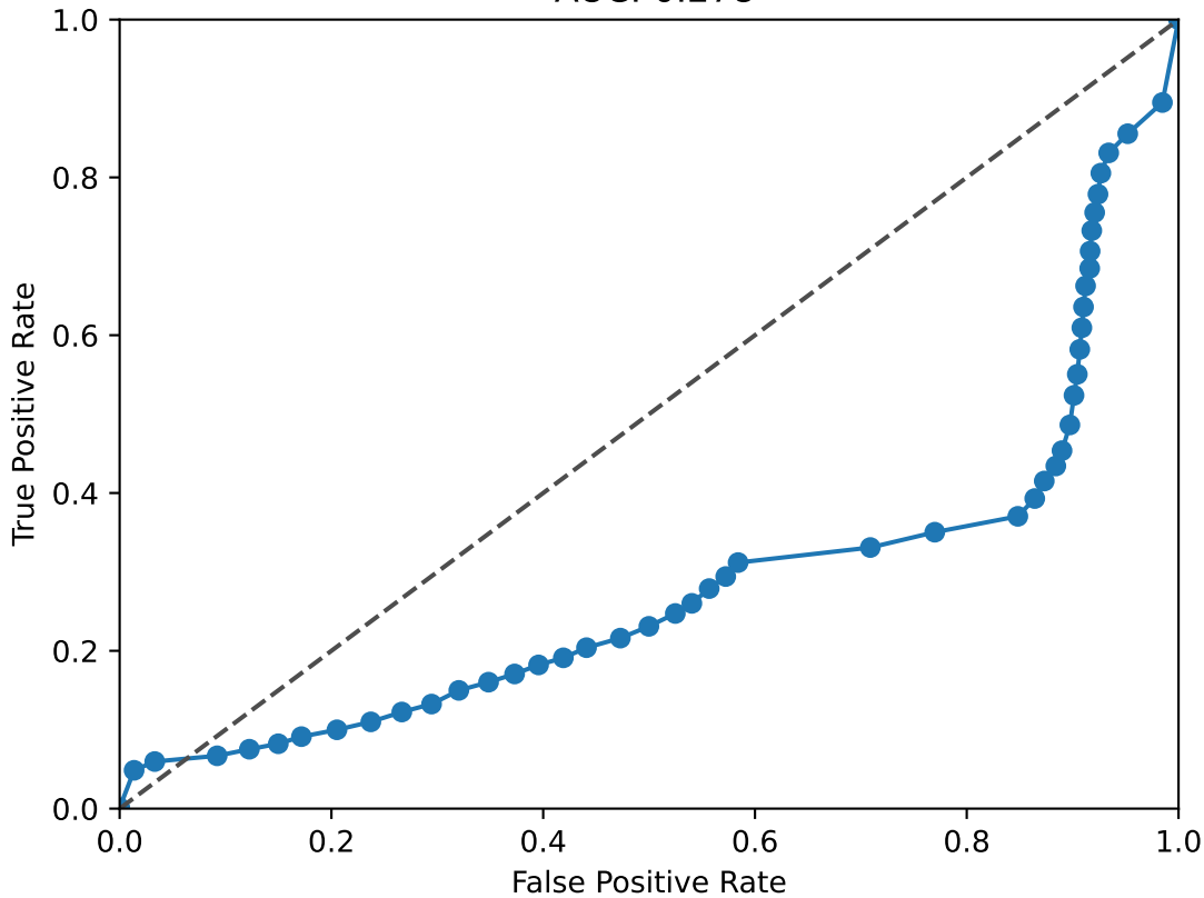
NFIA ROC Curve AUC: 0.278
