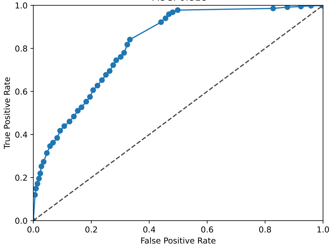
BACH2 ROC Curve AUC: 0.818
