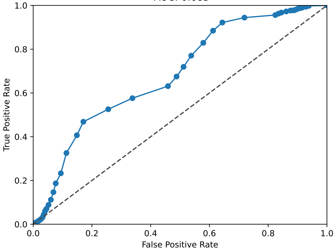
NFIA ROC Curve AUC: 0.685
