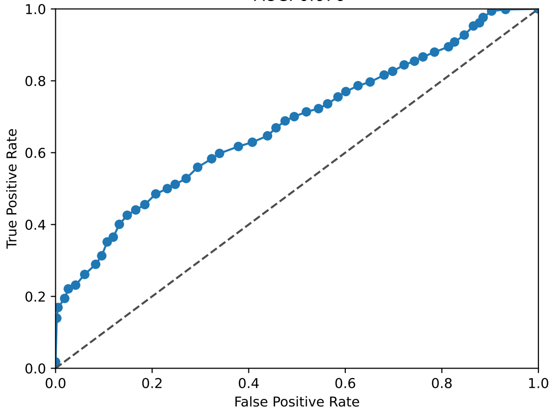
ZBTB20 ROC Curve AUC: 0.676
