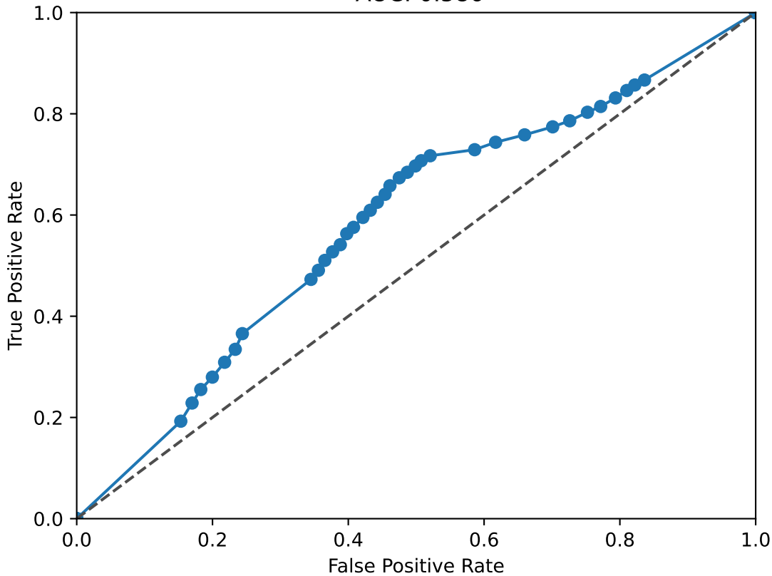
EHF ROC Curve AUC: 0.586
