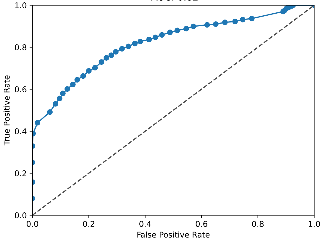
LMX1B ROC Curve AUC: 0.82
