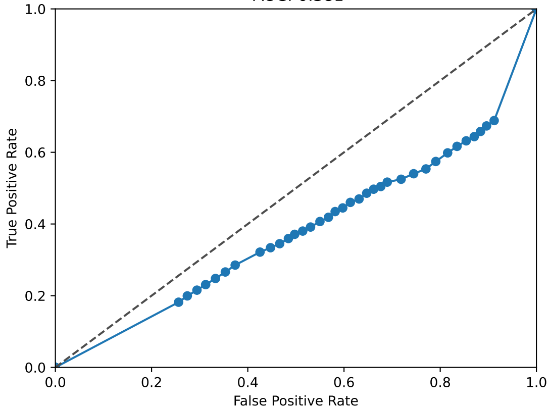
EHF ROC Curve AUC: 0.381
