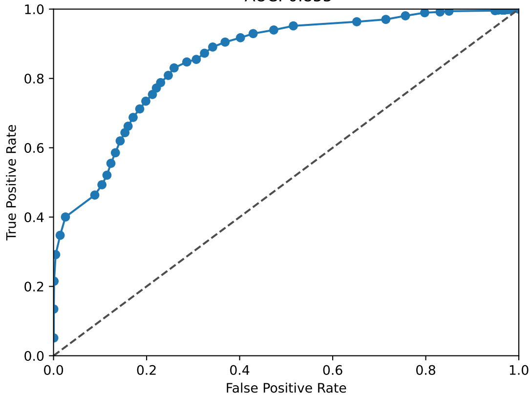
LMX1B ROC Curve AUC: 0.855
