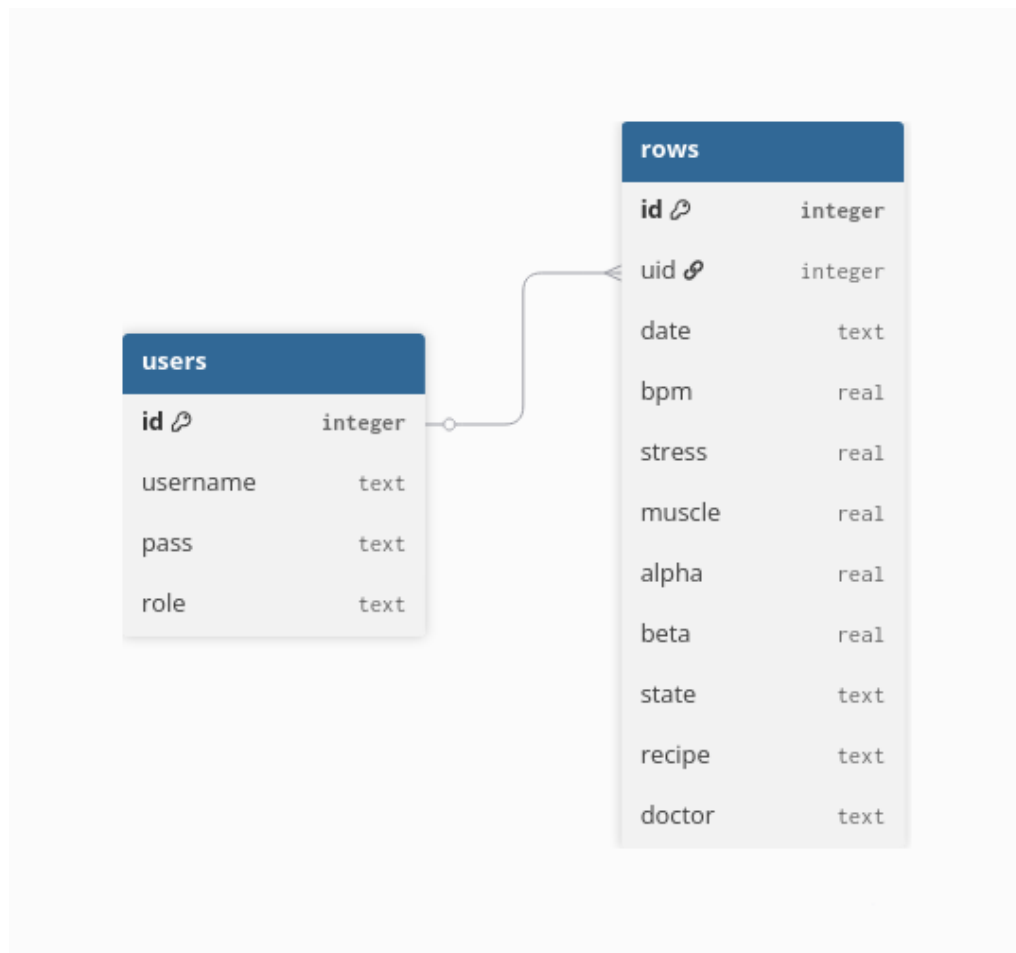
Рисунок 8 – ERD-схема базы данных проекта «Чумной Доктор»
