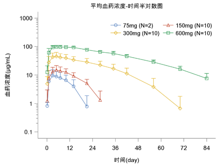
图 3: 健康受试者单次皮下注射 MG-K10 人源化单抗注射液后平均血药浓度-时间半对数 (Mean+SD) (PKCS)
