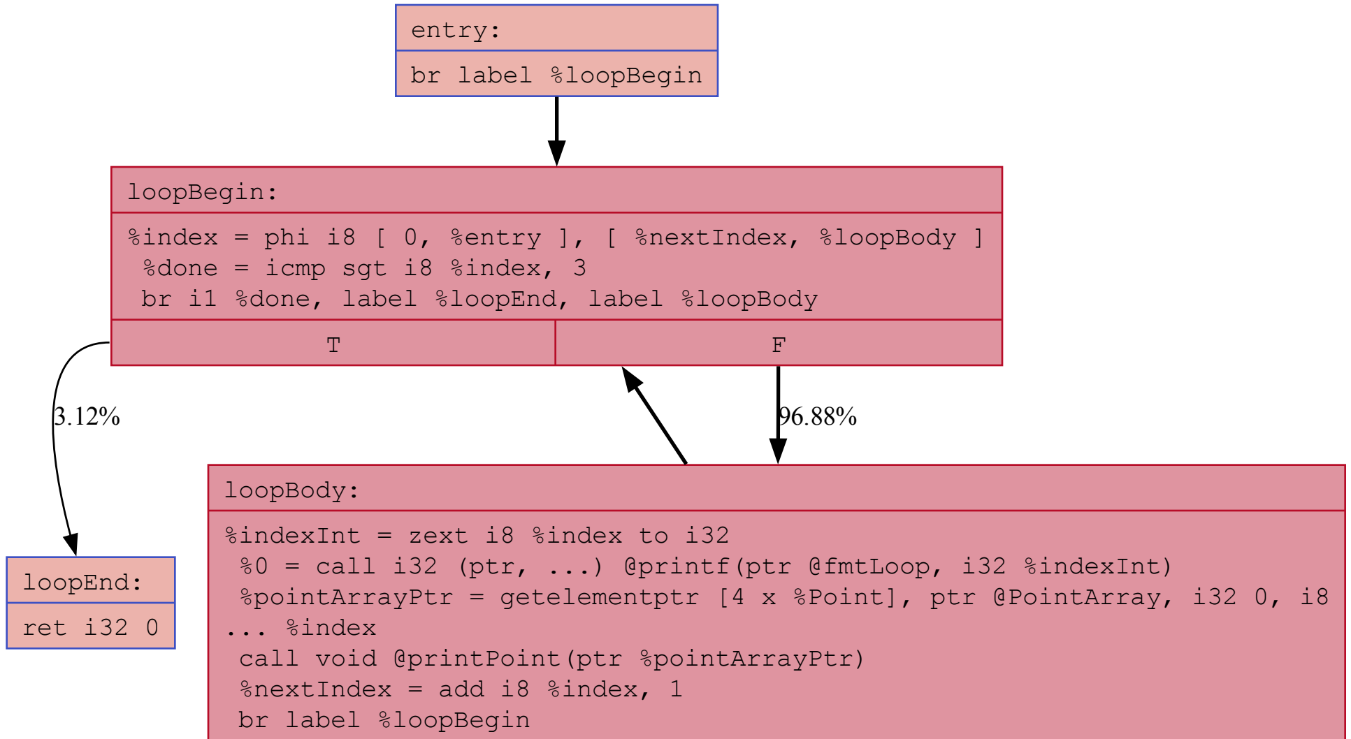
CFG for 'main' function
