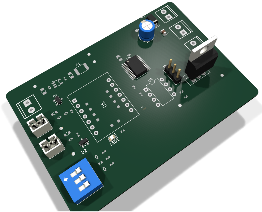
Figura 3: Vista isométrica del PCB v4. Se aprecian el DIP switch y conectores JST al borde izquierdo, el electrolítico de 48 V, el TB6612FNG (SSOP-24) y el MOSFET TO-220 en el dominio de potencia.
