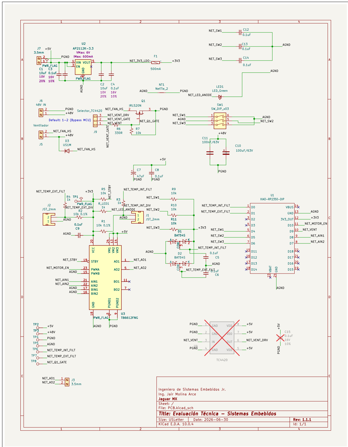
Figura 1: Esquemático del sistema (KiCad). Exportado directamente del proyecto.
