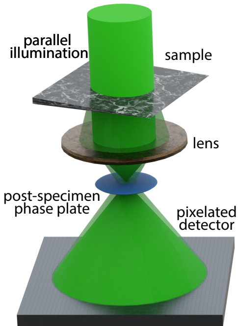
TEM phase contrast imaging
