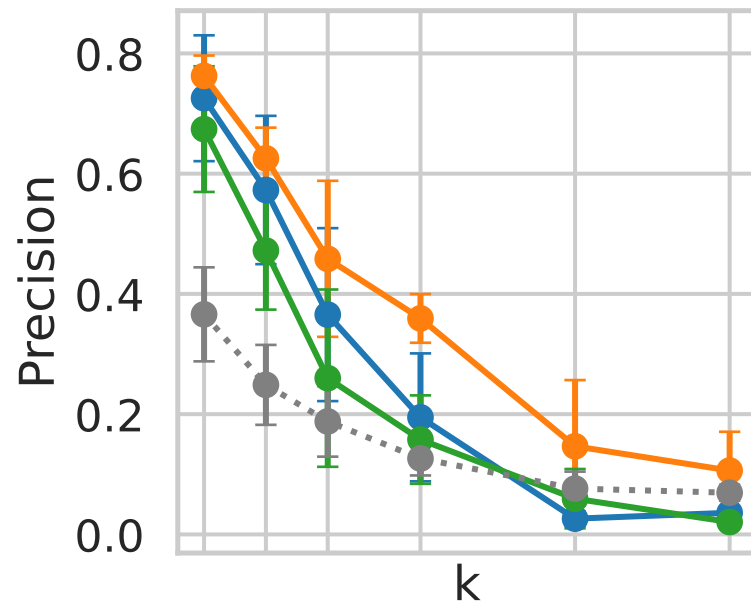
Precision
