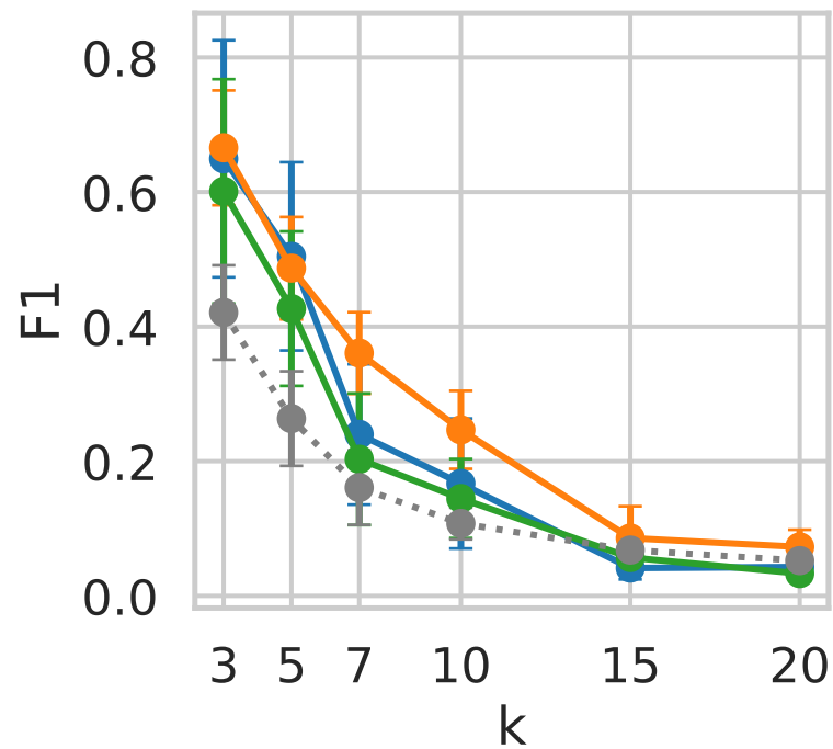
F1
