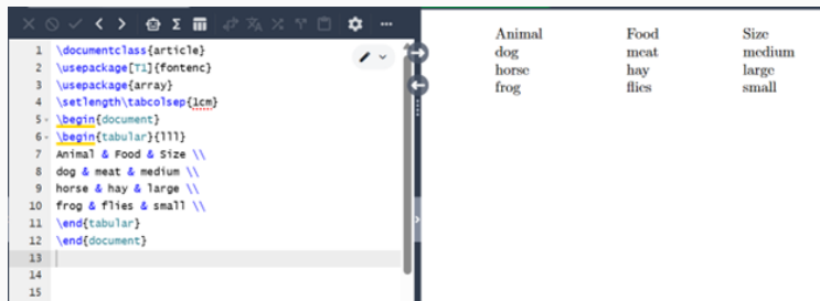
Рис. 10: LaTeX
