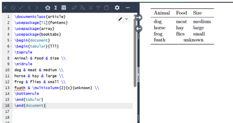
Рис. 7: LaTeX
