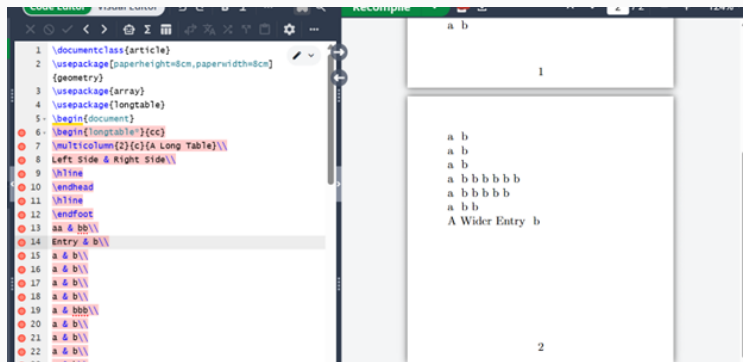
Рис. 13: LaTeX
