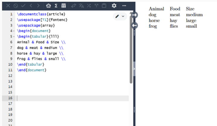
Рис. 1: LaTeX
