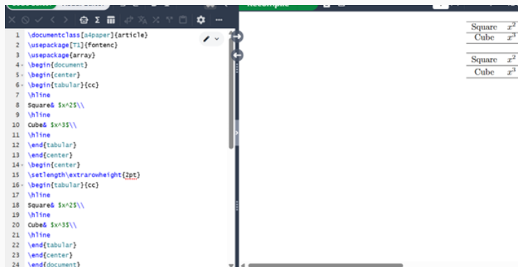
Рис. 15: LaTeX
