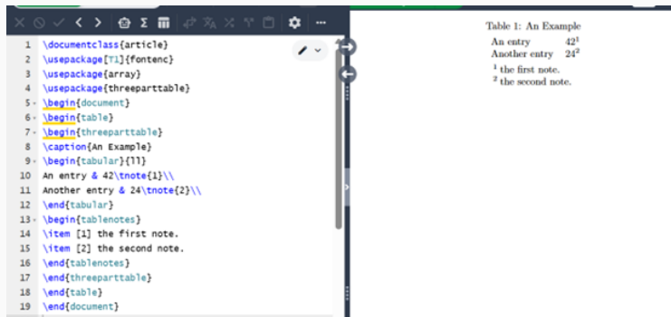
Рис. 14: LaTeX
