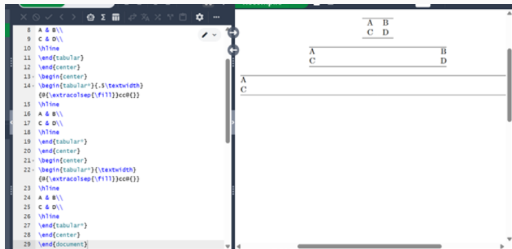
Рис. 12: LaTeX
