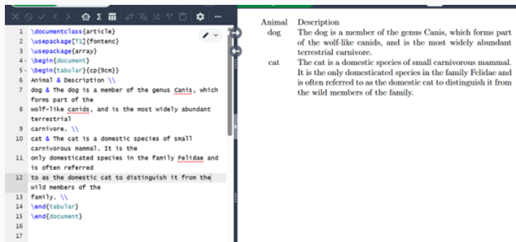
Рис. 3: LaTeX
