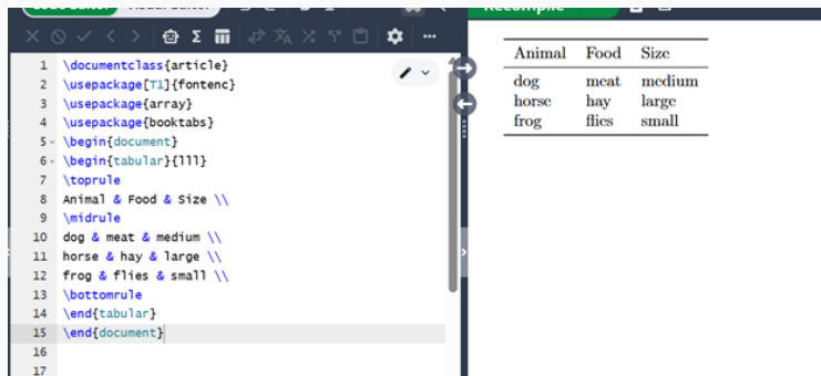
Рис. 5: LaTeX
