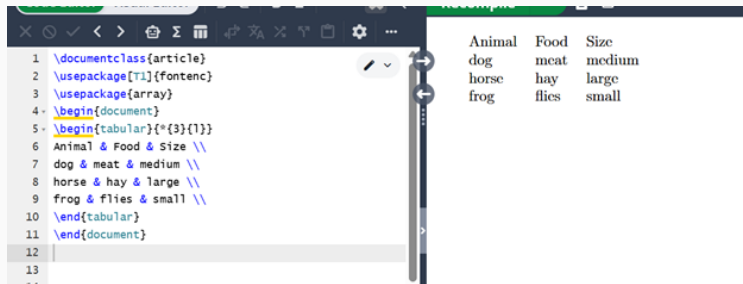
Рис. 4: LaTeX
