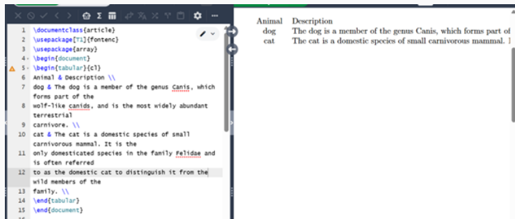
Рис. 2: LaTeX
