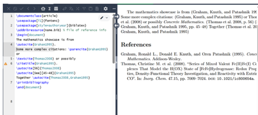
Рис. 3: Программа 3
