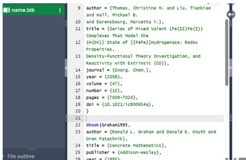
Рис. 1: Программа 1
