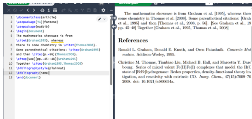
Рис. 2: Программа 2
