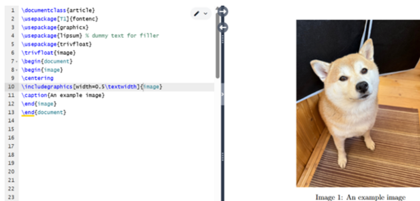
Рис. 6: Программа 6
