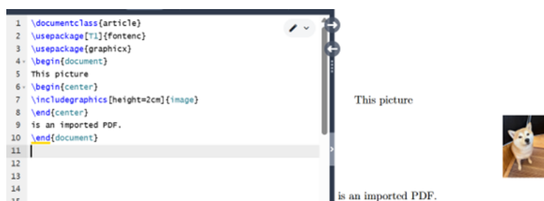
Рис. 1: Программа 1
