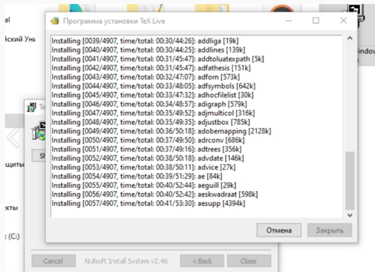
Рис. 1: LaTeX
