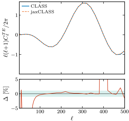
Cross C_\ell^{TE} \times 10^{-11}
