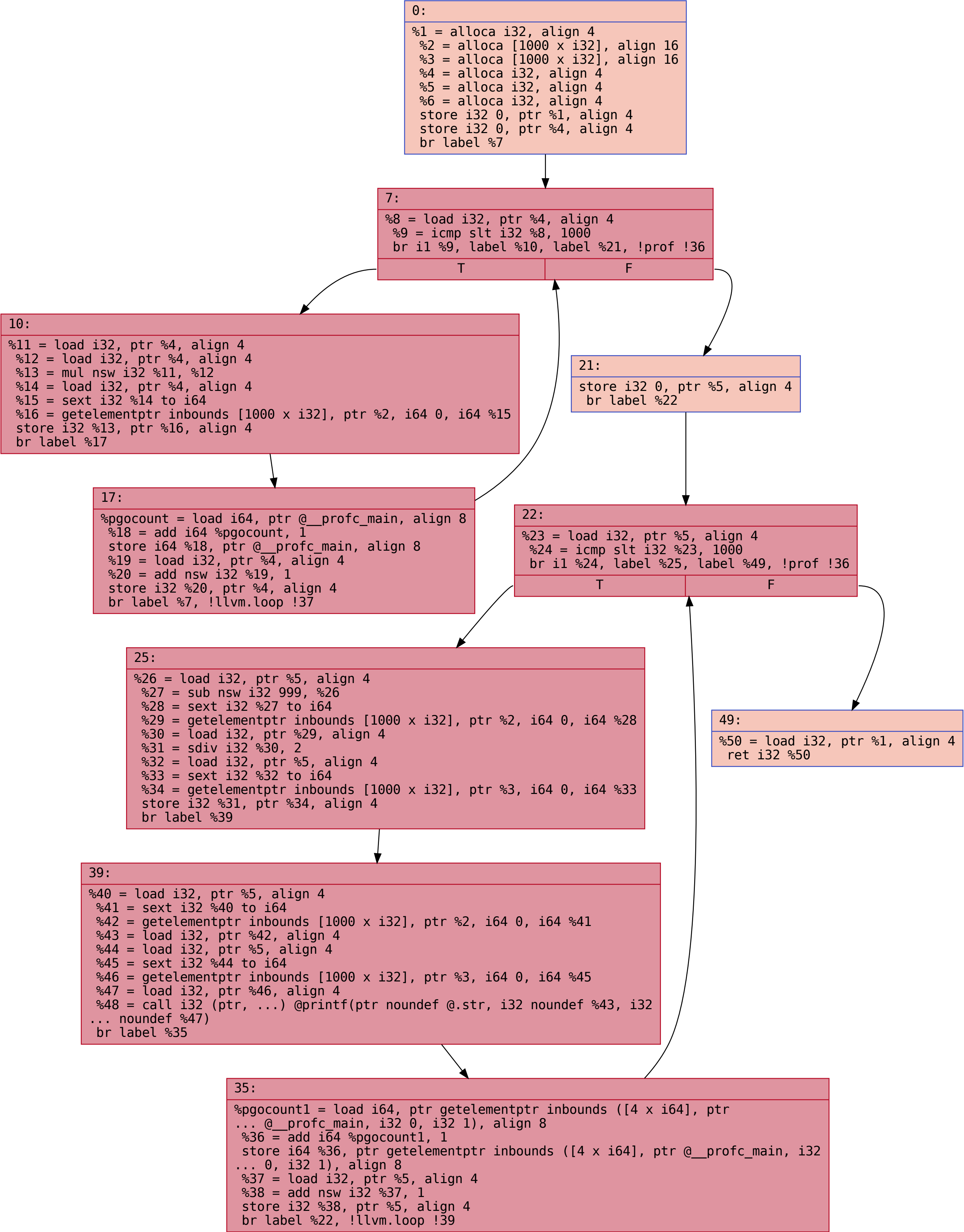
CFG for 'main' function
