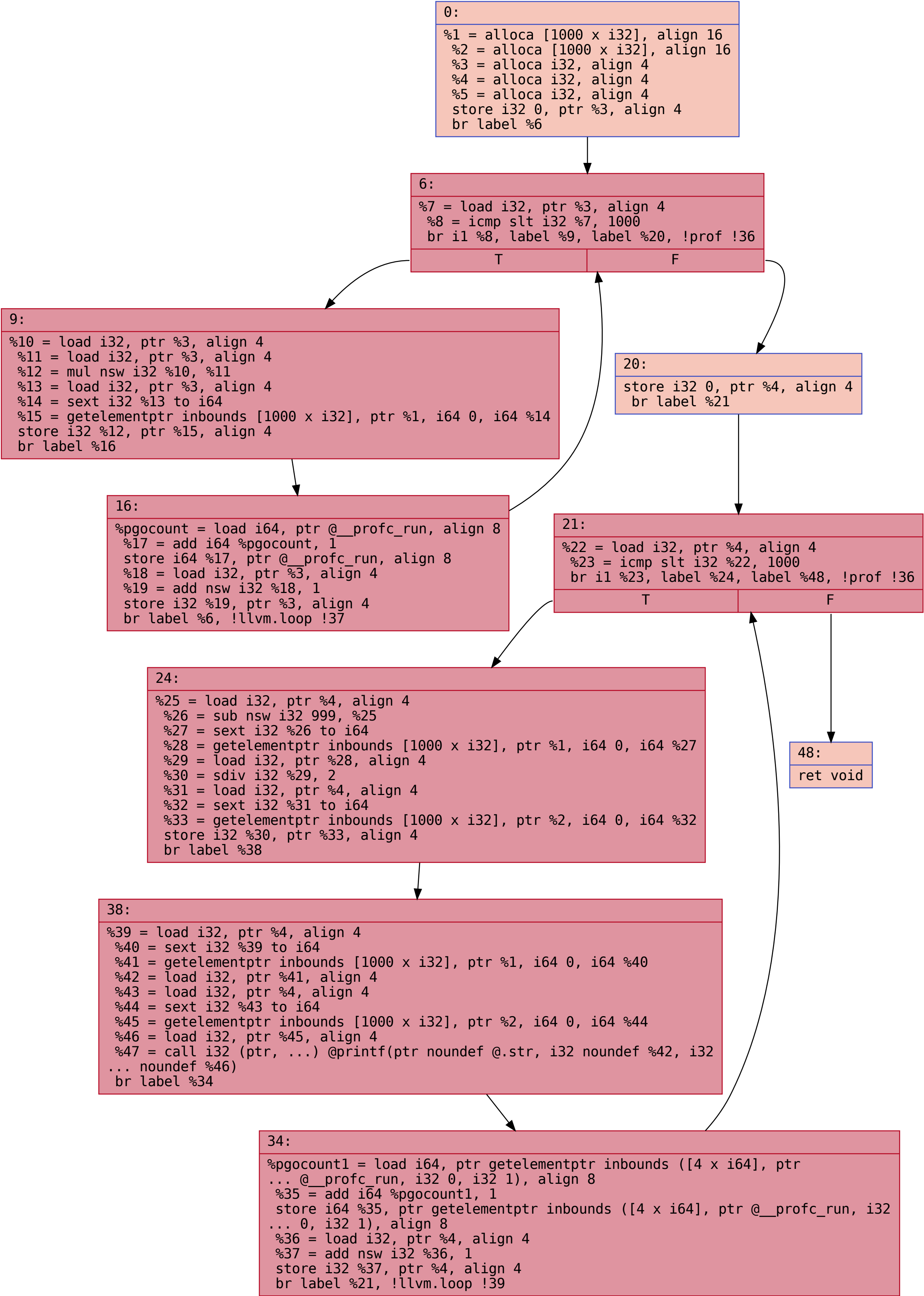
CFG for 'run' function
