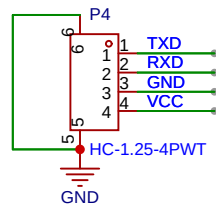
UART
