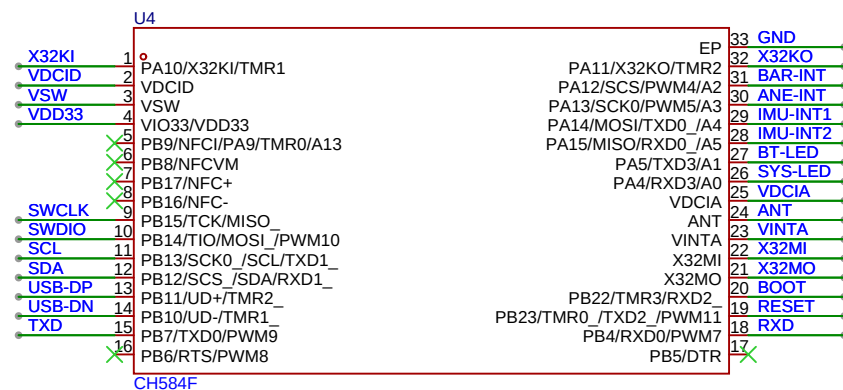
MCU
