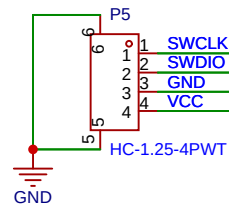
Debug
