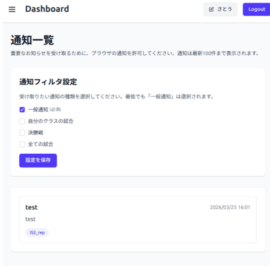
図 9 通知画面
