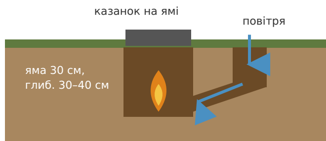
Рис. 10.2. Дакотське вогнище: дві ями, з'єднані тунелем. Майже без диму і світла, мінімум дров, сильна тяга
