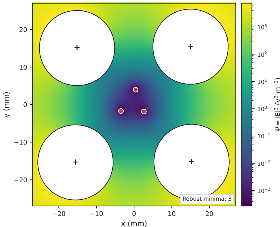
(d) In-phase connection: effective potential
