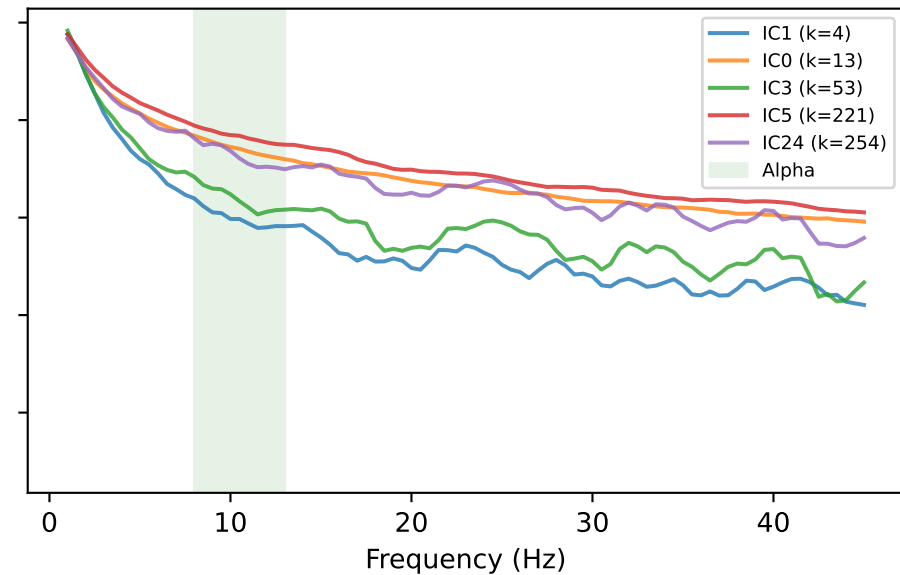
Infomax
