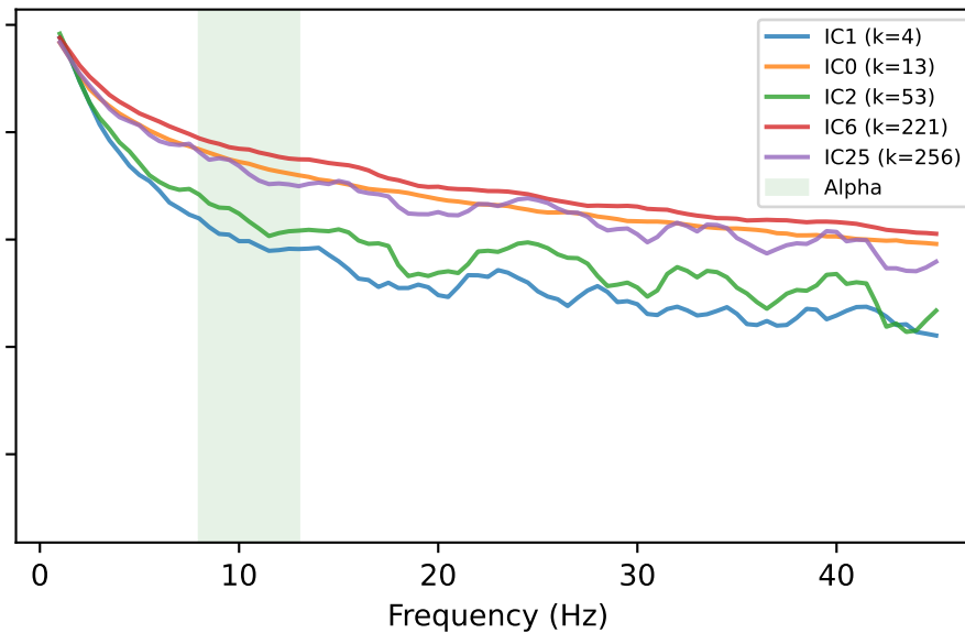
Picard
