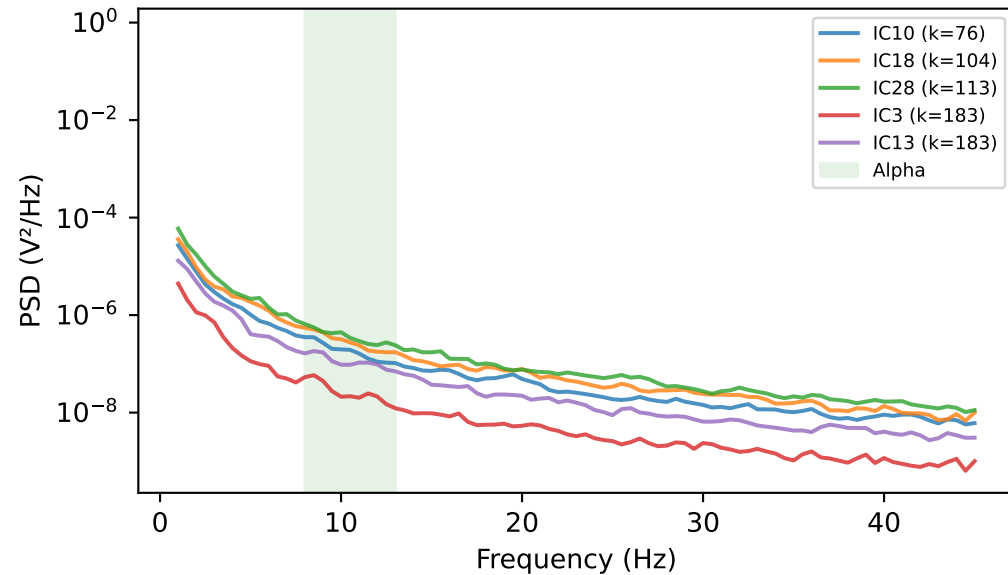
AMICA
