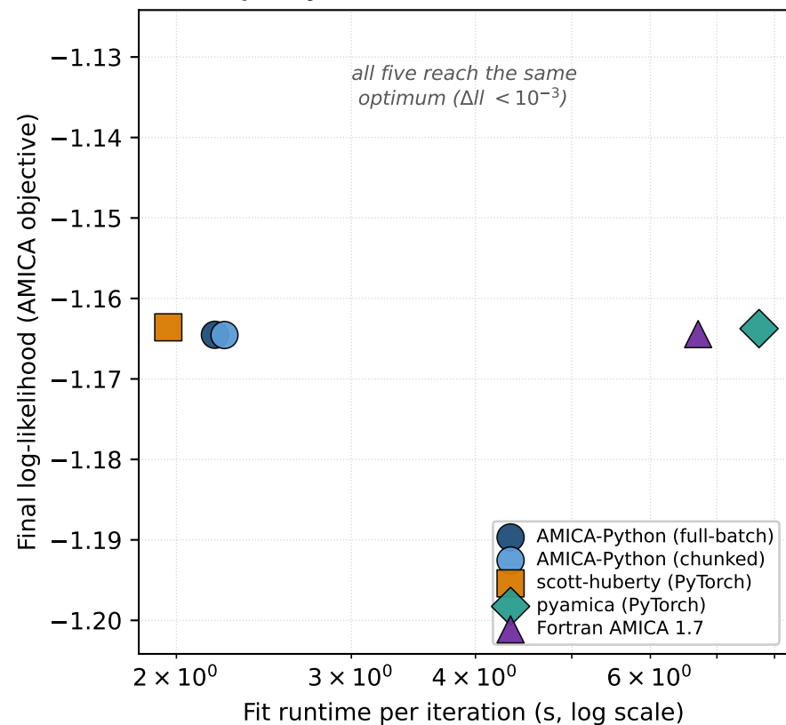
A. CPU quality-cost (sub-01)
