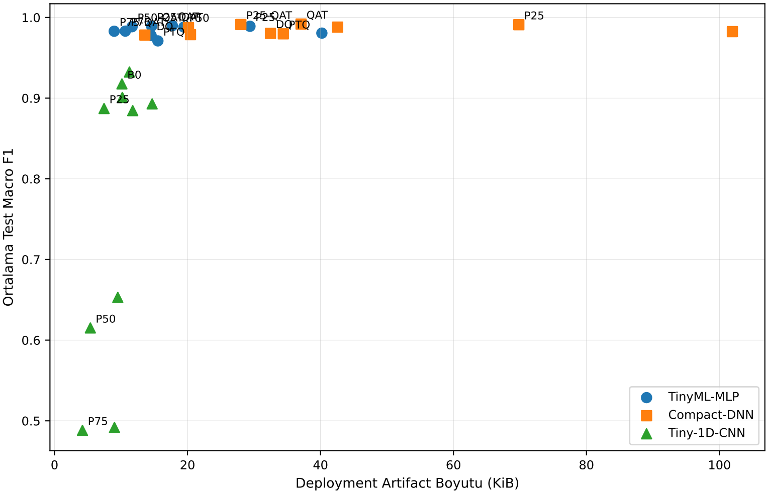
Doğruluk-Model Boyutu Ödünleşimi
