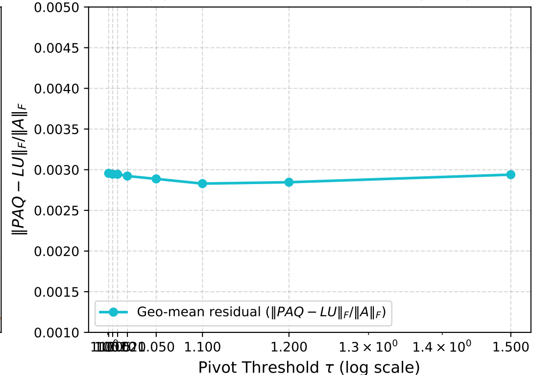
(d) Numerical Invariance Across \tau ( w = 6 )
