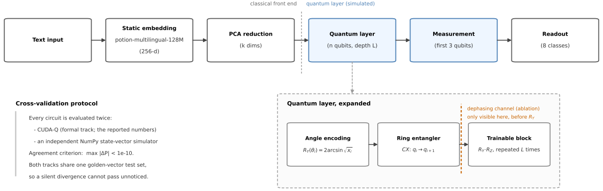
图 1: 系統架構。古典前端（靜態嵌入 → 主成分分析 principal component analysis, PCA 降維）輸出 k 維特徵，交給量子層：角度編碼 R_Y(\theta_i) = 2 \arcsin \sqrt{x_i} 、環形 CX 糾纏、可訓練的 R_Y \times R_Z 區塊重複 L 次；量測只取前 3 個 qubit（ 2^3 = 8 個基底模式，與 n 、 L 無關），再由古典讀出層映射到 8 個類別。左下角為交叉驗證協定；展開框標出相位消融的插入位置——必須在含 R_Y 的層之前，否則量測不到任何效果（實測機率變化 1.4 \times 10^{-17} ）。
