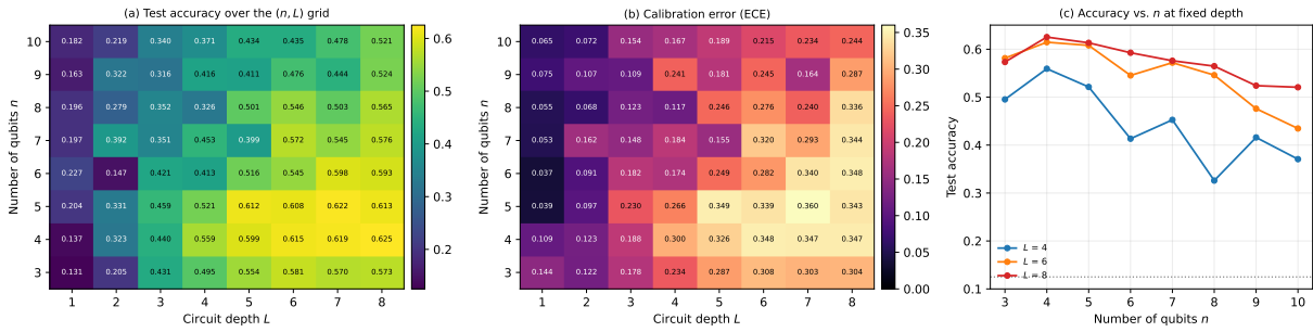
图 2: (n, L) 網格上的測試準確率與校準誤差（5 個種子的平均值）。面板 (a)(b) 為熱圖，格子內的數字為精確值，淺灰格表示尚未執行；面板 (c) 為固定深度切面，直接檢驗準確率對 qubit 數的依賴。
