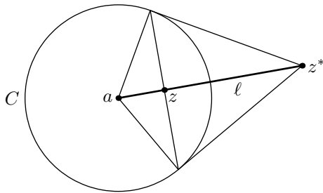
図 3.38 反転
