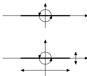
図 2.44 C_2 と D_2
