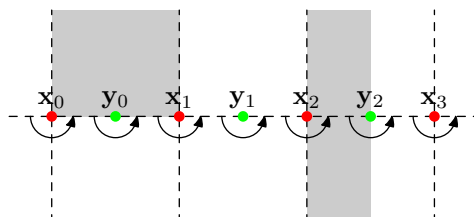
図 2.46 F_2
