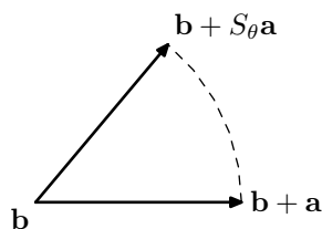
図 2.18 ST_{\mathbf{a}}S^{-1}
