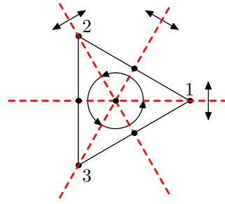
図 A.15 D_3
