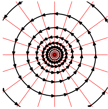
図 3.58 図 3.43 再掲
