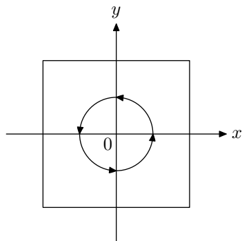
図 1.11 巡回群 C_4
