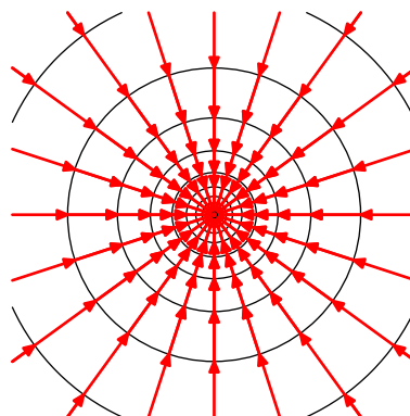
図 3.45 双曲型
