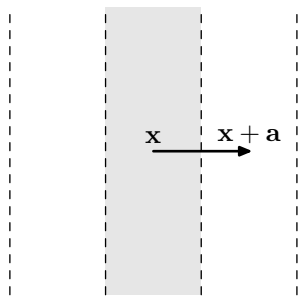
図 2.92 F_1
