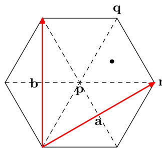
図 2.33
