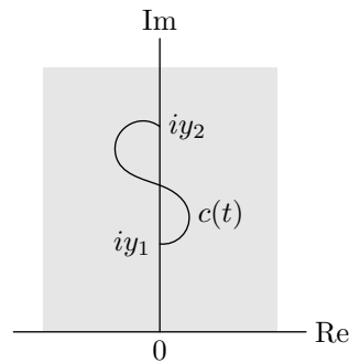
図 3.65 H^+ と曲線
