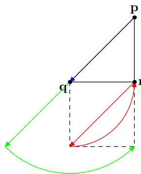
図 2.36
