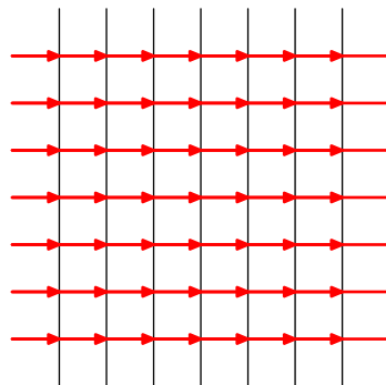
図 3.47 放物型
