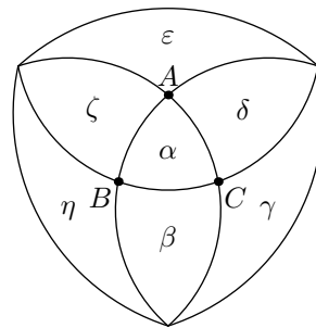
図 3.53 模式図
