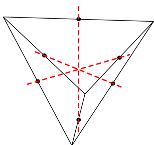
図 1.21 \pi 回転
