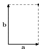
図 2.52 長方形格子
