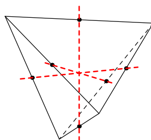
図 1.22 \pi 回転
