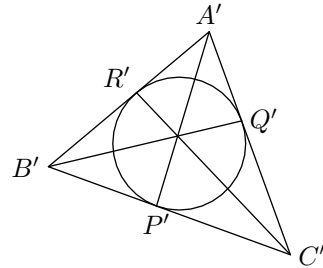
図 3.22 内接円
