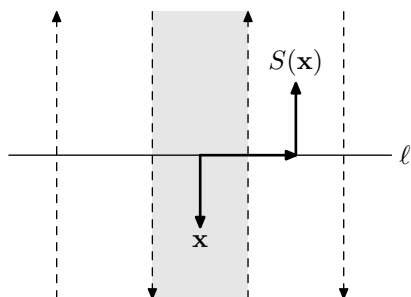
図 2.94 F_2
