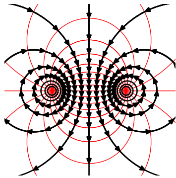
図 3.60 図 3.42 再掲
