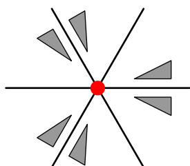
图 2.84 D_3, 0, D_5 , 万华镜
