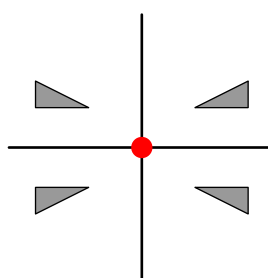
图 2.83 D_2, 0, D_2 , 万华镜
