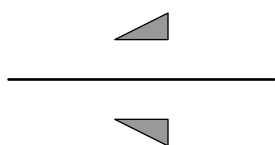
图 2.82 D_1, 0, D_1 , 万华镜
