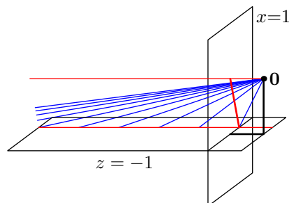
図 3.7 直線の射影
