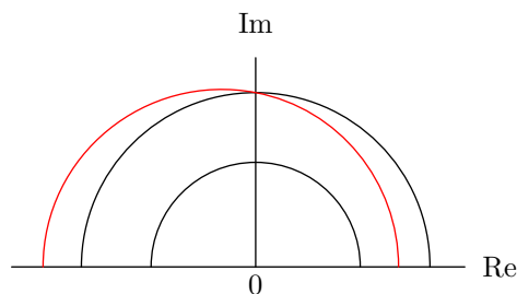
図 3.73 \mathbf{H}^+ での直線の様子
