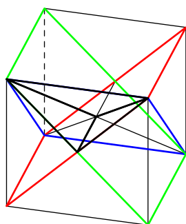
図 3.64 シンプルルート \bullet \xrightarrow{3} \bullet
