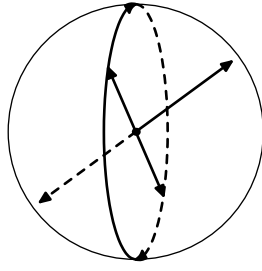
図 3.29 実射影平面 P^2
