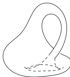
図 2.99 \mathbf{R}^3 のクラインの壺
