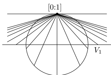
図 3.31 \mathbf{P}^1 と S^1
