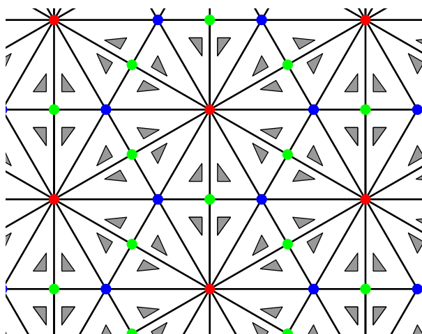
图 2.72 P6mm , 正六角形, D_6 , 万华镜
