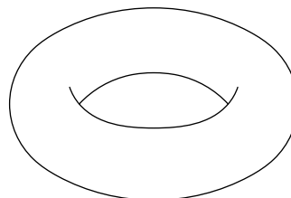
図 2.93 \mathbb{R}^3 のトーラス
