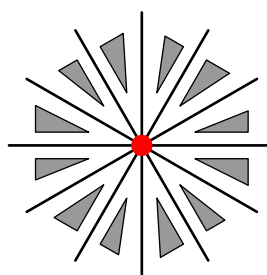
图 2.83 D_6, 0, D_6 , 万華鏡
