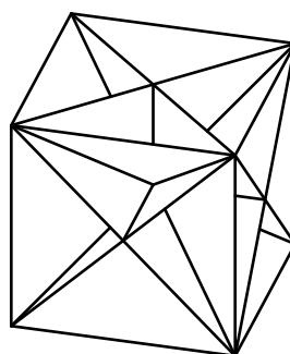
図 3.65 立方体の分割
