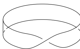
図 2.91 \mathbb{R}^3 のメビウスの帯
