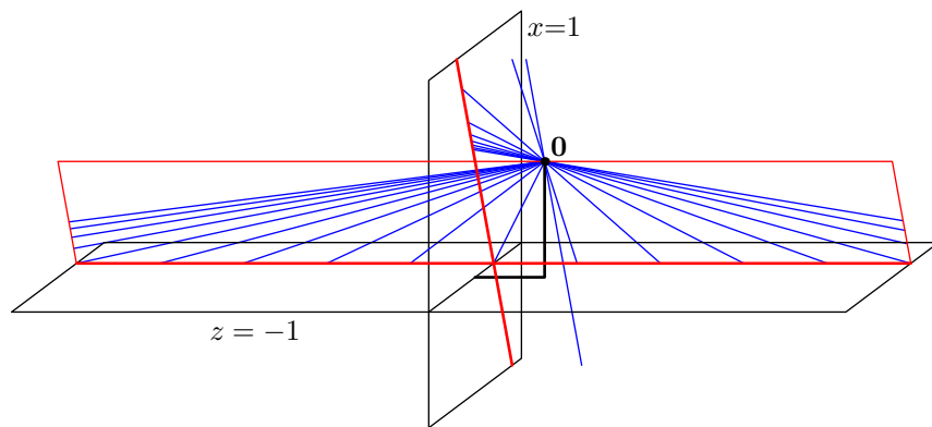
図 3.25 後ろからの透視投影
