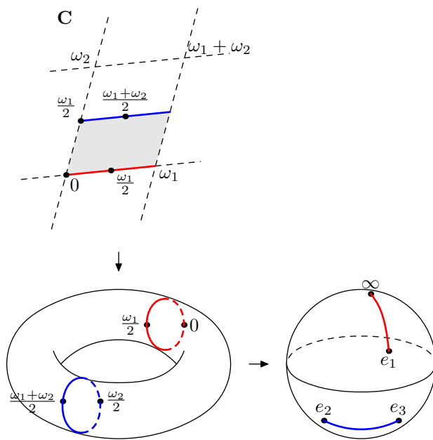
図 3.80 P : T \rightarrow \mathbf{CP}^1 \simeq S^2
