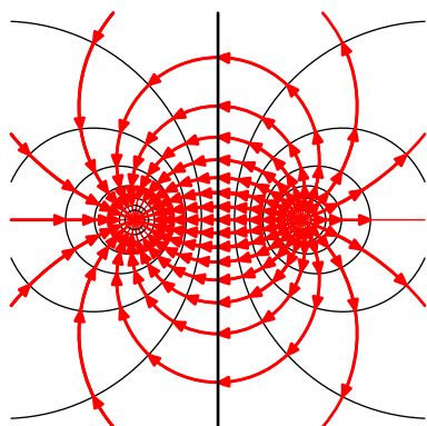
図 3.44 双曲型
