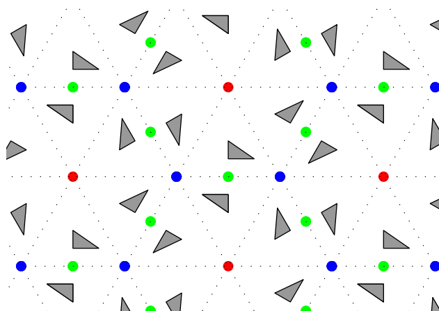
图 2.71 P6 (M5) , 正六角形, C_6
