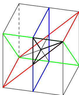
図 3.62 シンプルルート \bullet \xrightarrow{4} \bullet
