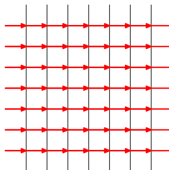
図 3.47 放物型
