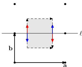
図 2.98 平坦クラインの壺
