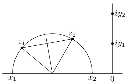
図 3.72 \mathbf{H}^+ の測地線
