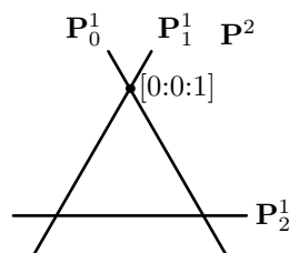
図 3.32 \mathbf{P}^2 と \mathbf{P}_0^1, \mathbf{P}_1^1, \mathbf{P}_2^1
