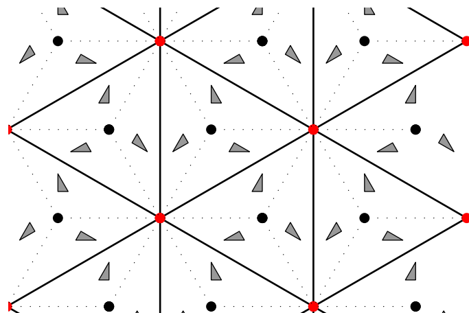
图 2.70 P31m , 正六角形, D_3
