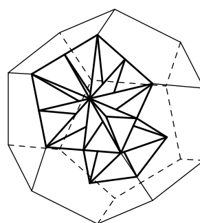
図 3.67 正 12 面体の分割の一部
