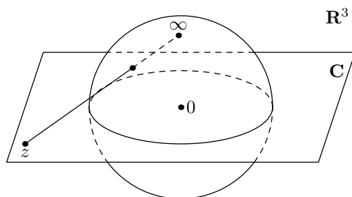
図 3.36 リーマン球面
