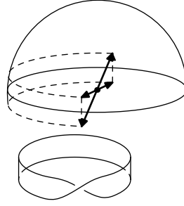
図 3.30 P^2 とメビウスの帯
