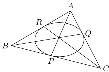
図 3.21 ジュルゴンヌ点
