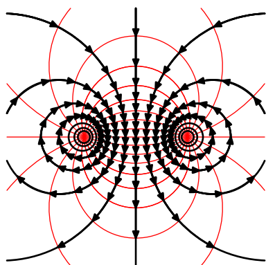
図 3.42 楕円型
