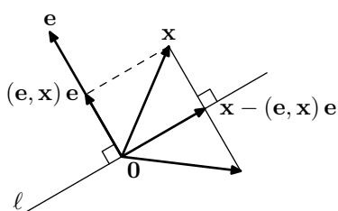
図 1.3 直線 \ell での鏡映
