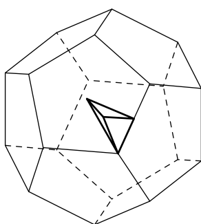
図 3.66 シンプルルート \bullet \xrightarrow{5} \bullet
