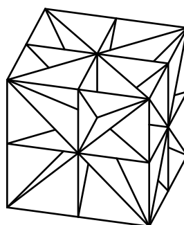
図 3.63 立方体の分割
