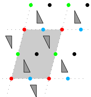
図 2.57 P2 (M_2) , 一般, C_2
