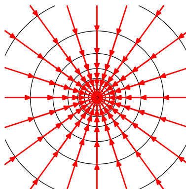
図 3.45 双曲型
