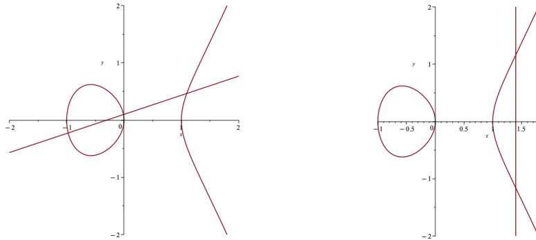
図 3.78 虚軸に平行でない直線との 図 3.79 虚軸に平行な直線との交点 交点 P + Q + R = O P + P' = O
