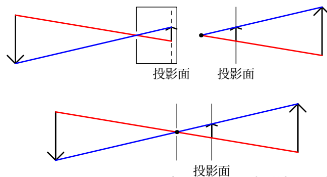
図 3.26 カメラ・オブスキュラと遠近法の融合
